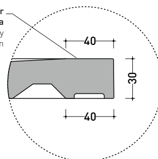
dettaglio del bordo / shower tray rim detail
