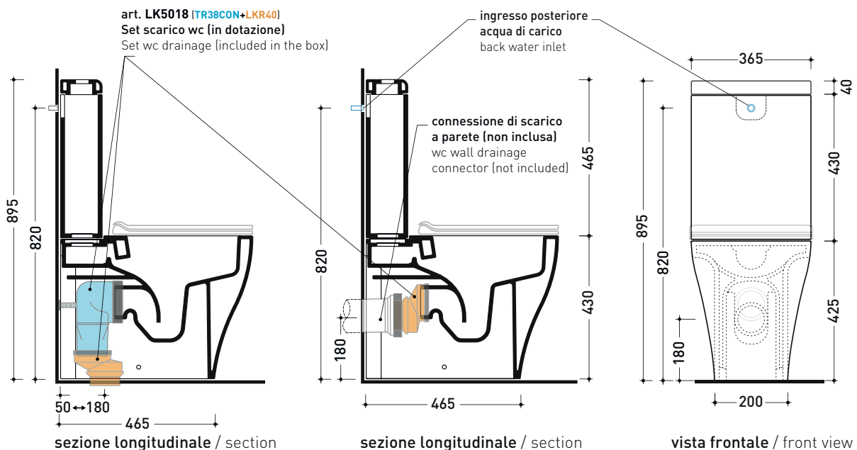
sezione longitudinale / section
