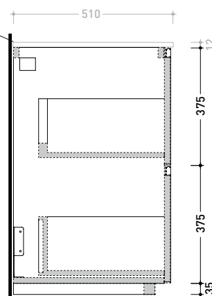
sezione
