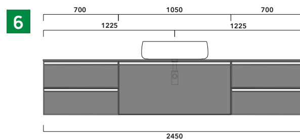
6 | profondità cm 50: n.2 CKD425 + n.1 CKD893 + CKPR51 cm 245
