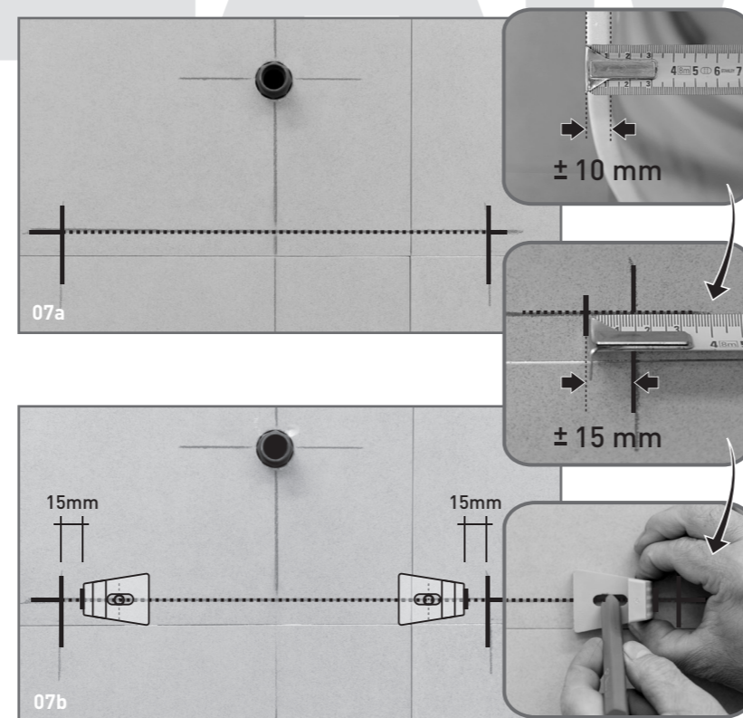
07 Preparazione al fissaggio delle staffe: tracciare l'allineamento dei fori di fissaggio (07a); rilevare lo spessore della ceramica ( \pm 10 mm) riportare la misura maggiorata ( \pm 15 mm) sulla parete; quindi con la staffetta in plastica segnare la posizione dei fori per il fissaggio. Preparation for fastening the brackets: mark the alignment of the fixing holes (07a); measure the thickness of the ceramic urinal ( \pm 10 mm) and mark out the increased measurement ( \pm 15 mm) on the wall; then use the plastic bracket to mark the position of the fixing holes.
