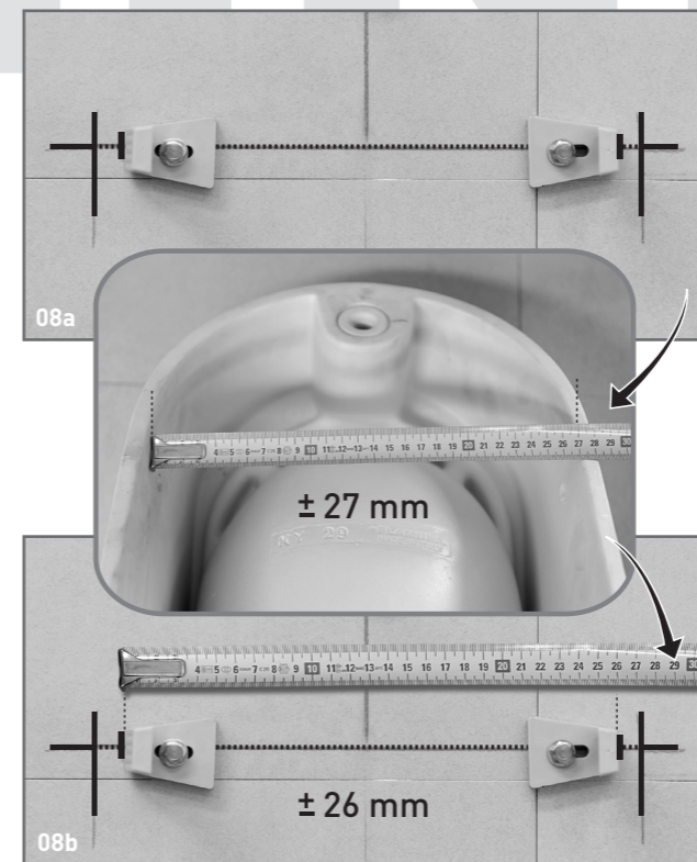
08 Fissaggio delle staffe: bloccare le due staffe come da foto (08a). Rilevare la misura interna del sanitario ( \pm 27 mm) e successivamente verificare che la distanza fra le staffe sia inferiore di circa 10 mm ( \pm 26 mm) a quella rilevata. Dopodichè serrare bene le staffe nella posizione corretta. Fixing of the brackets: block the two brackets as shown in the photo (08a). Measure the inside of the sanitary fixture ( \pm 27 mm) and then check that the distance between the brackets is at least 10mm ( \pm 26 mm) less than the measurement. Securely fasten the brackets in the correct position.
