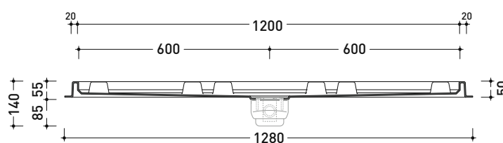
sezione trasversale / section
