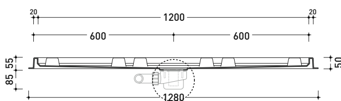
sezione longitudinale / section
