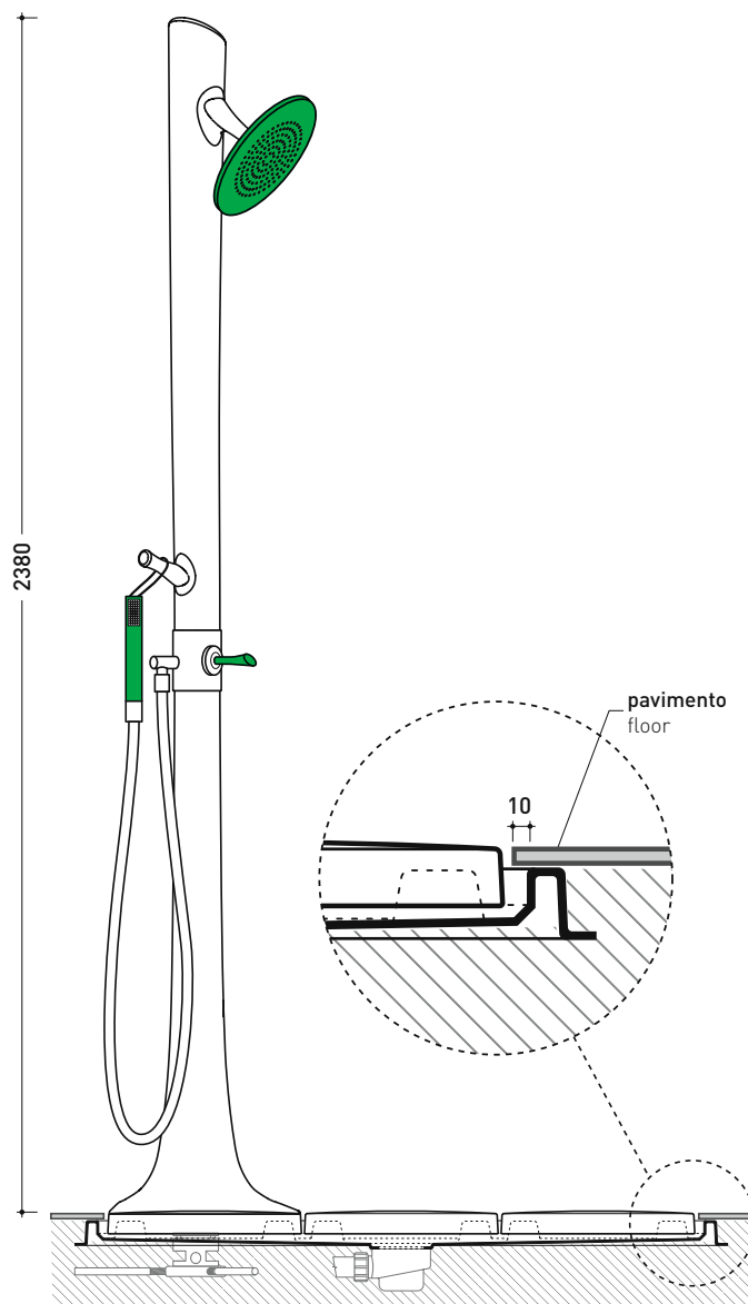
sezione longitudinale / section
