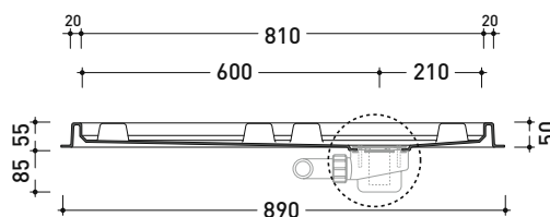
sezione longitudinale / section
