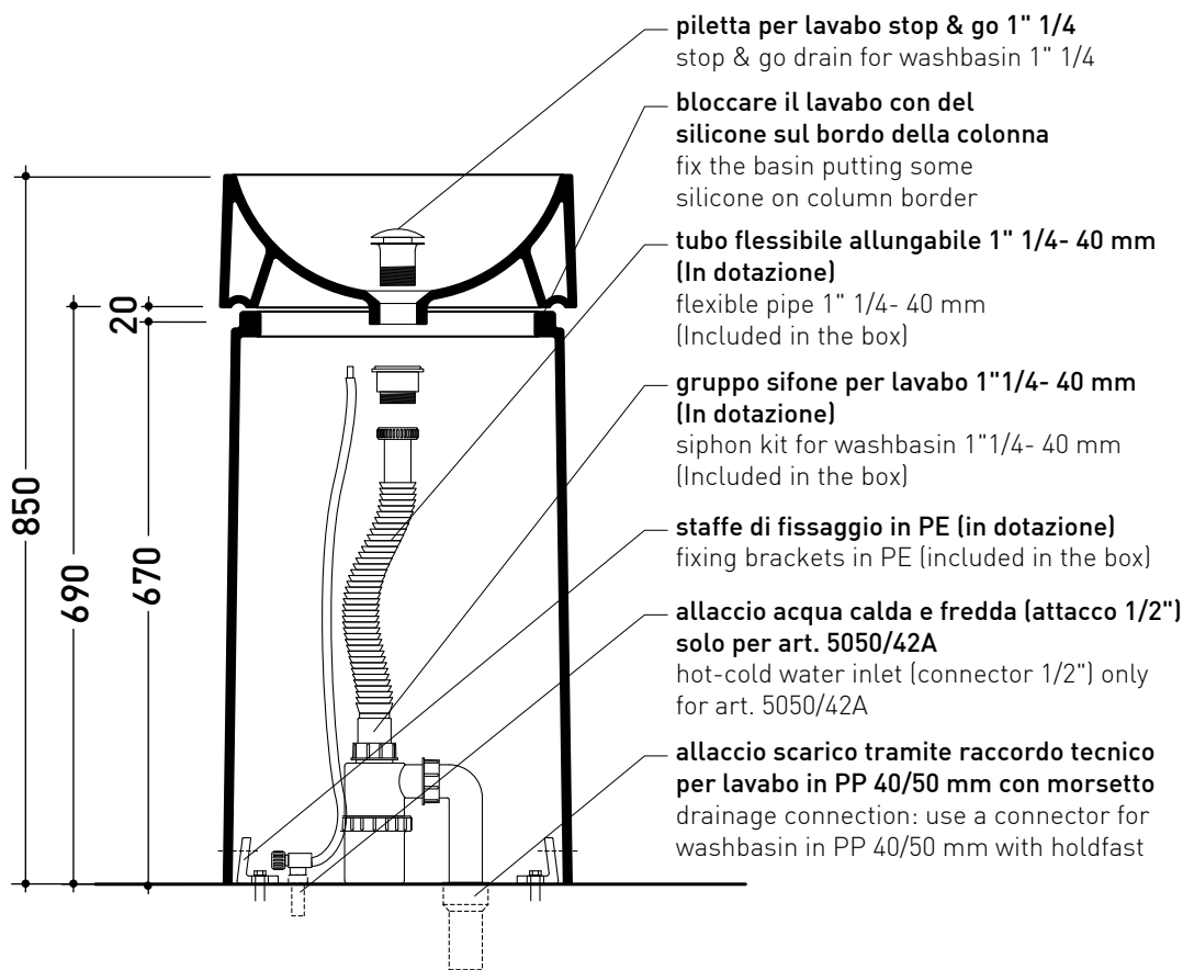
sezione longitudinale / section
