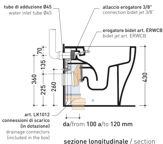
sezione longitudinale / section
